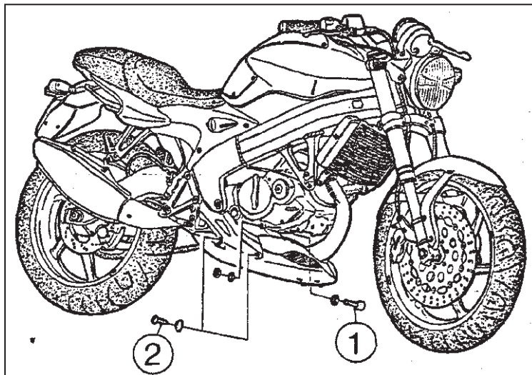
FIG. 17 1. Vite fissaggio carenatura 2. Vite fissaggio carenatura
