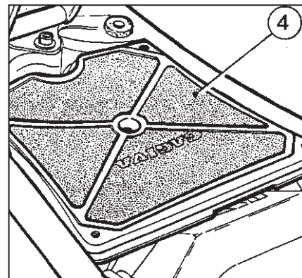
FIG. 24 4. Elemento filtrante
