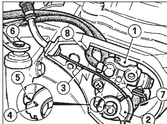
FIG. 14 POMPA OLIO
