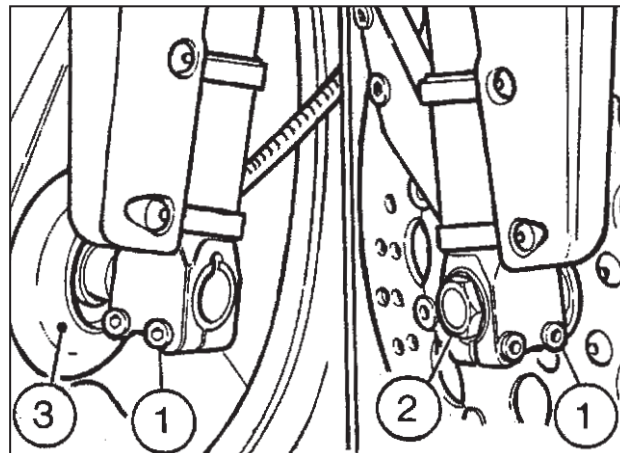
BILD 35 1. Feststellschraube für den Zapfen 2. Radzapfenmutter 3. Kilometerzählers
