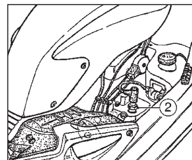
Fig. 25 1- Vite fissaggio pannello 2- Candela accensione
