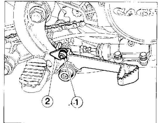
1) Dado / Nut / Ecrou / Mutter / Tuerca 2) Piastrina di registro pedale / Pedal adjustment plate / Plaque réglage pedale / Pedaleinstellplättchen / Placa de regulación pedal
