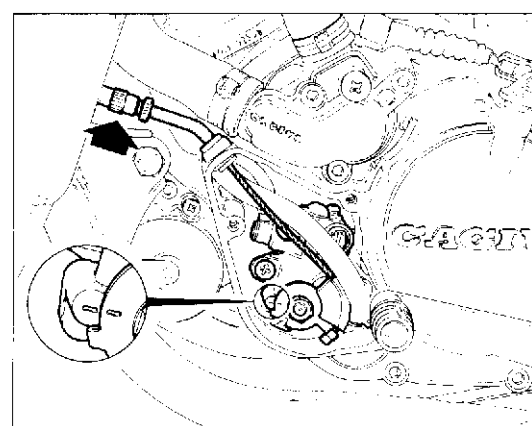
1) Coperchio pompa olio / Oil pump cover / Couvercle pompe à huile / Ölumpendeckel / Tapón bomba aceite.
