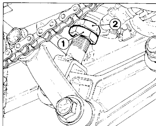
1) Controdado / Lock nut / Contre-écrou / Gegenmutter / Contra-tuerca 2) Dado di registro / Register nut / Ecrou de registre / Regelmutter / Tuerca de ajuste
